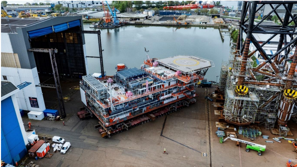
Productieplatform N05-A in aanbouw
